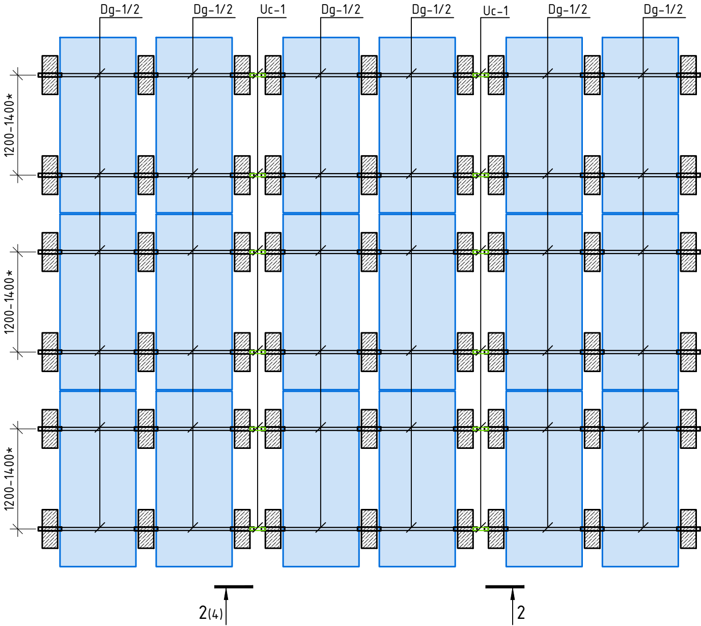
Система кріплення SRS-B-Lite-EW. Фрагмент для 18 ФЕМ
